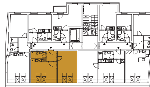
Schéma půdorys
