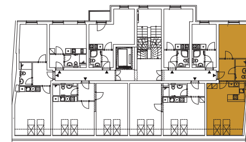
Schéma půdorys
